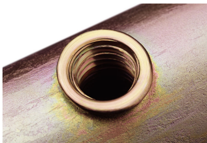
Flowdrill® på runde rør, buede profiler og hvælvede overflader giver en helt plan anlægsflade.
